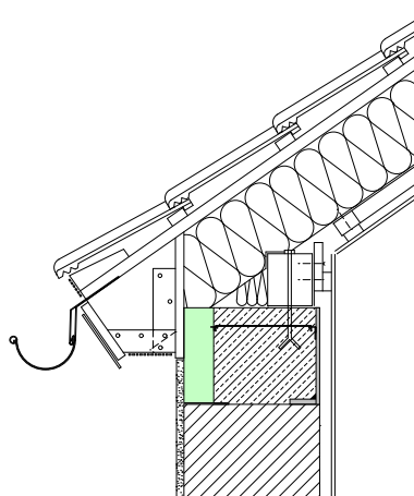
Monolithische Wandkonstruktion
