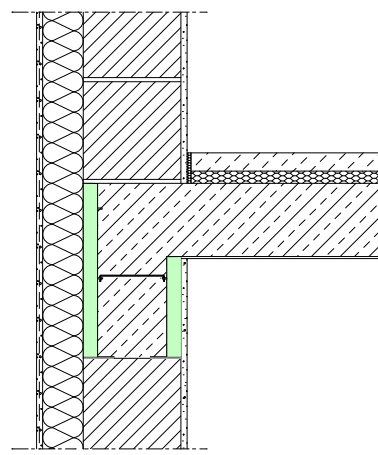
WDVS Wandkonstruktion
