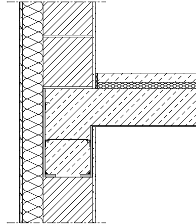
WDVS Wandkonstruktion
