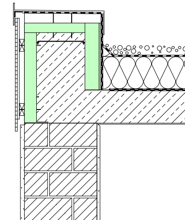
Monolithische Wandkonstruktion
