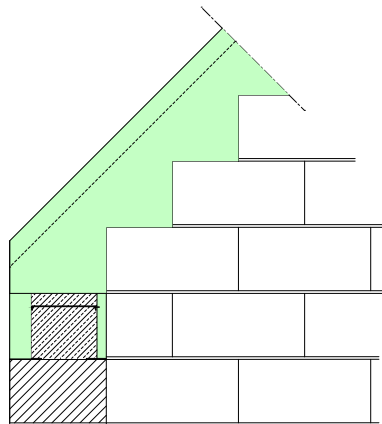
Giebelansicht
