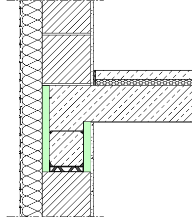
WDVS Wandkonstruktion
