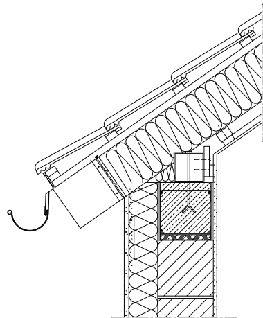
WDVS Wandkonstruktion
