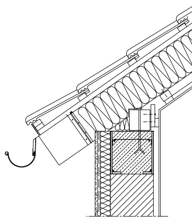
WDVS Wandkonstruktion
