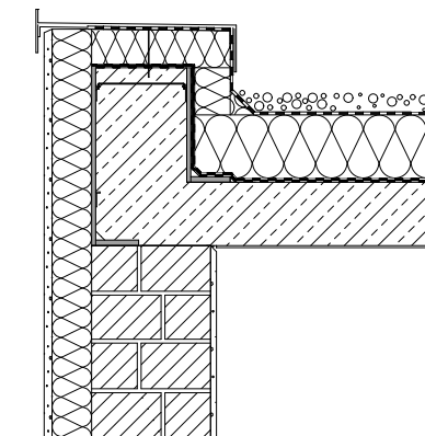
WDVS Wandkonstruktion
