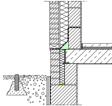
Mehrschalige Wandkonstruktion
