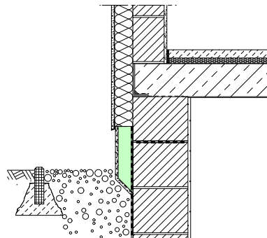
WDVS Wandkonstruktion
