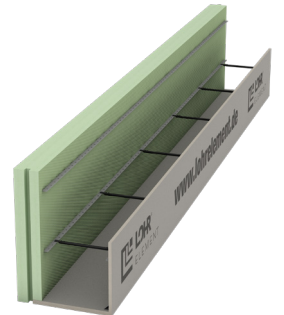
Typ SKE 80/F/F mit Ankerleiste mit Deckenrandabschalung
