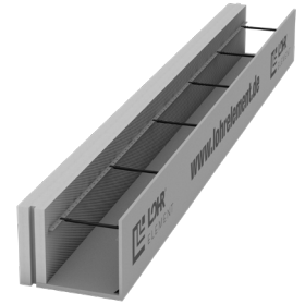
Typ SKE 80/F/F NH mit Ankerleiste
