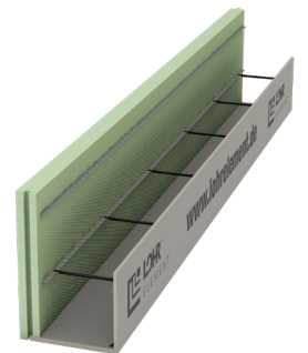
Typ SKE 60/F/F mit Ankerleiste mit Deckenrandabschalung
