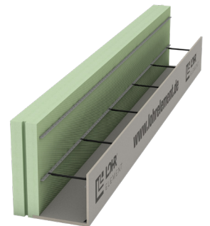
Typ SKE 120/F/F mit Ankerleiste mit Deckenrandabschalung
