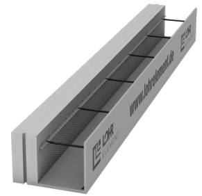
Typ SKE 120/F/F NH mit Ankerleiste
