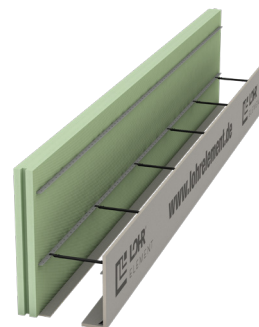
Typ RS 60/F mit Ankerleiste mit Deckenrandabschalung
