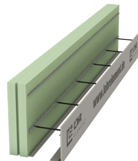
Typ RS 120/F mit Ankerleiste mit Deckenrandschalung
