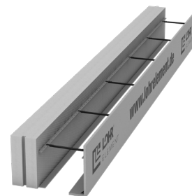
Typ RS 120/F NH mit Ankerleiste
