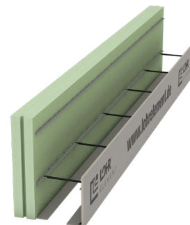
Typ RS 100/F mit Ankerleiste mit Deckenrandabschalung
