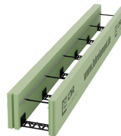
Typ MPA4 80/50 mit Ankerleiste
