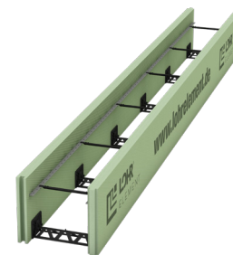
Typ MPA4 35/35 mit Ankerleiste
