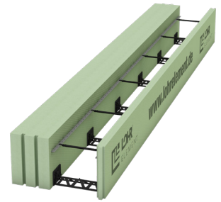
Typ MPA4 180/35 mit Ankerleiste
