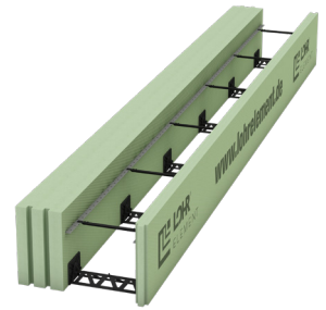
Typ MPA4 140/35 mit Ankerleiste
