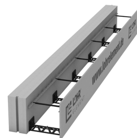
Typ MPA4 100/F NH mit Ankerleiste
