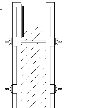
Stahlbetonwand
