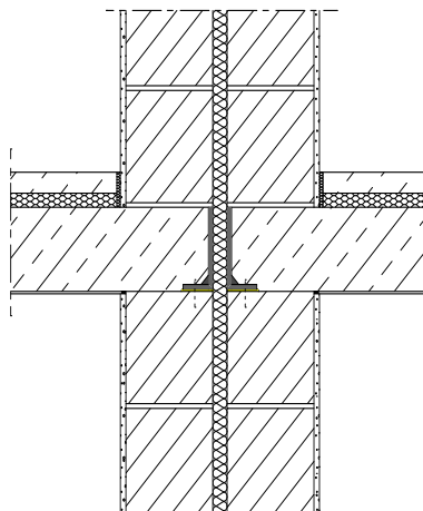
Haustrennwände
