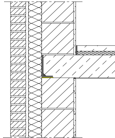
Mehrschalige Wandkonstruktion
