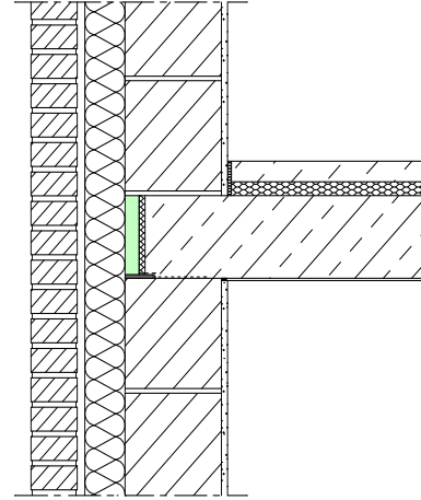
Mehrschalige Wandkonstruktion
