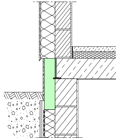
WDVS Wandkonstruktion
